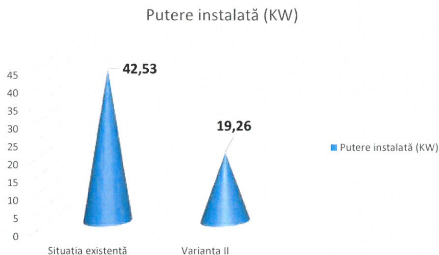
Fig. 14 Comparație putere totală instalată
