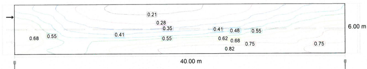
Observator 2: Densitatea luminii la instalația nouă [ \text{cd}/\text{m}^2 ] (Linii Isolux)
