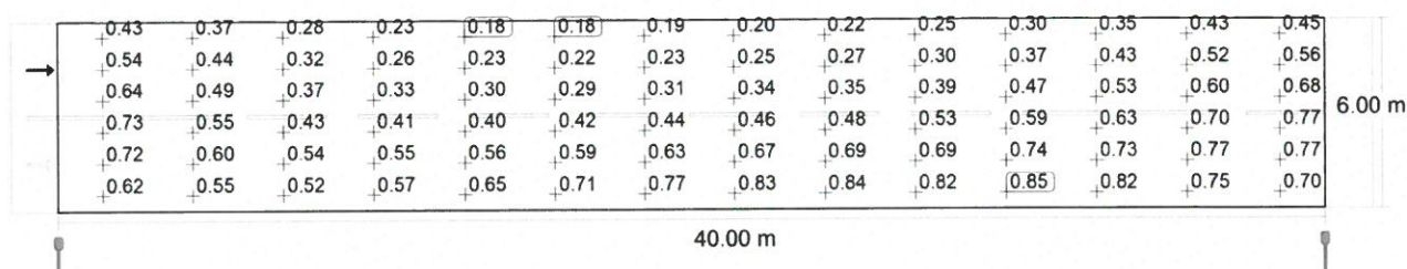
Observator 2: Densitatea luminii la instalația nouă [ \text{cd}/\text{m}^2 ] (Raster valoric)
